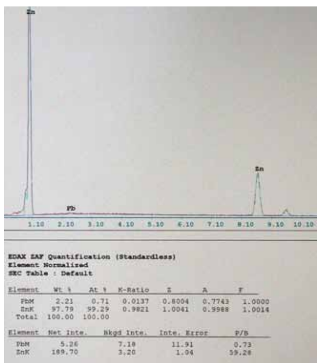
Výsledky plošné analýzy zinkové slitiny (SEM - EDX)
