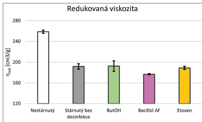
Obr. 2 Porovnání redukované viskozity pro dezinfikované vzorky a nedezinfikovaný standard / Comparison of reduced viscosity for disinfected samples and non-disinfected standard
